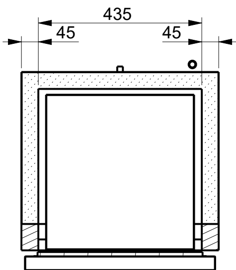
SEZIONE B-B
