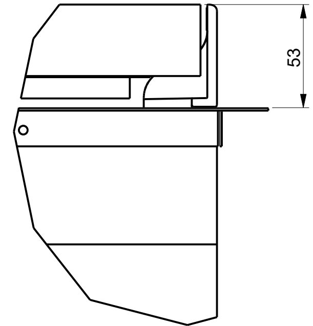
DETTAGLIO A CORNICE DI FISSAGGIO
